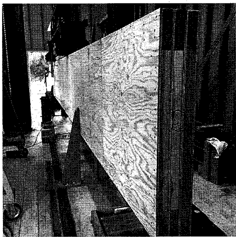
杉合成充複梁の構造実験(福岡県農林業総合試験場)
