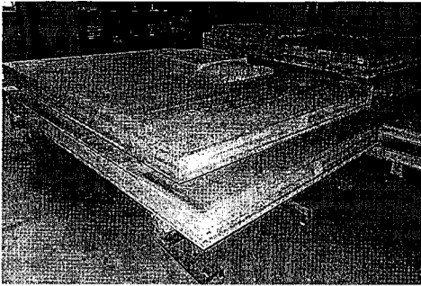
同社工場に加工されたCLT材
